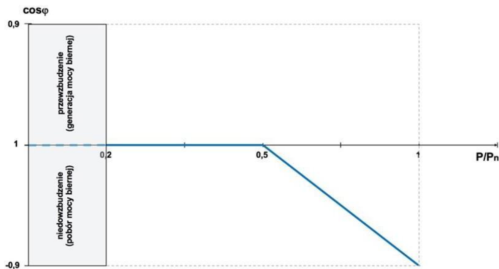
Rys. 5. Charakterystyka sterowania współczynnikiem mocy \cos \phi w funkcji generowanej mocy czynnej wymagana przez OSDn
